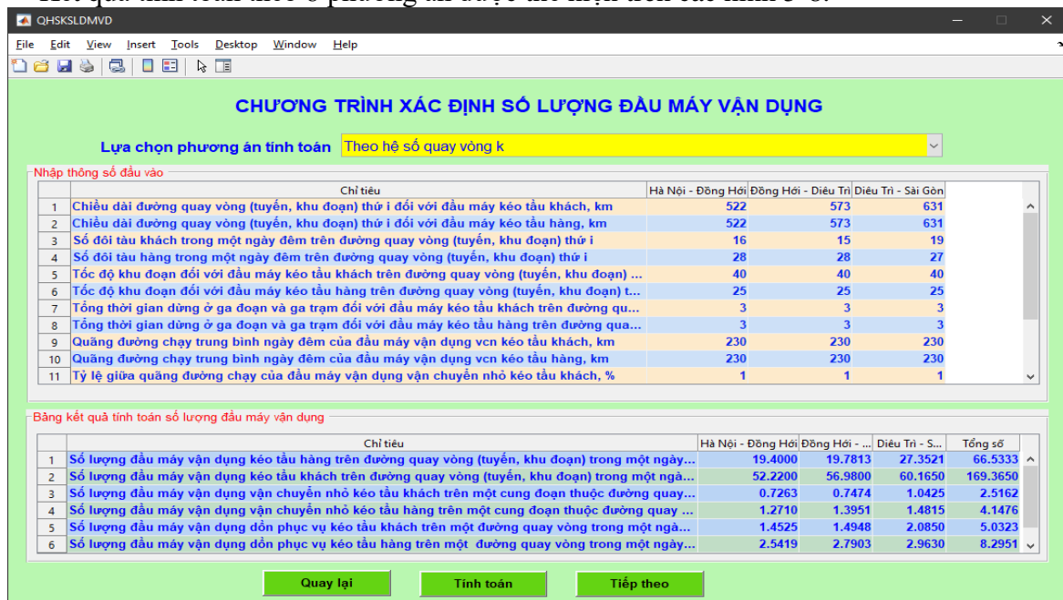
Hình 5. Giao diện chương trình tính toán xác định số lượng đầu máy vận dụng trên tuyến Hà Nội - Sài Gòn theo phương án A1 ( k=1,15 ).
