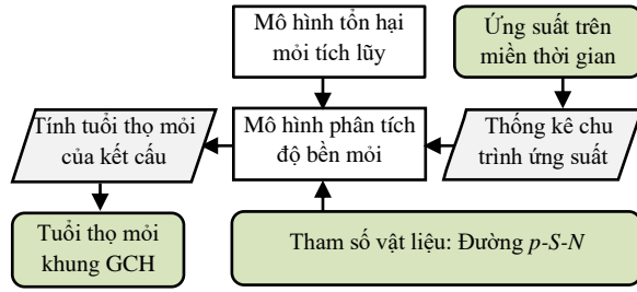
Hình 8. Mô hình phân tích độ bền mỏi
