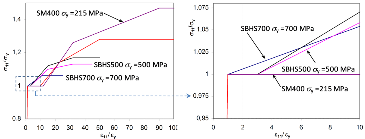
Hình 12. Đặc tính vật liệu của các cấp thép trong phạm vi 2 \varepsilon_y .
