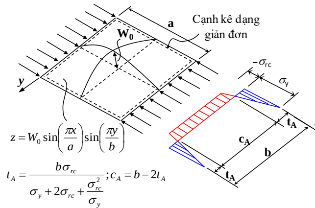
Hình 3. Mô hình kết cấu của tấm thép khảo sát.
