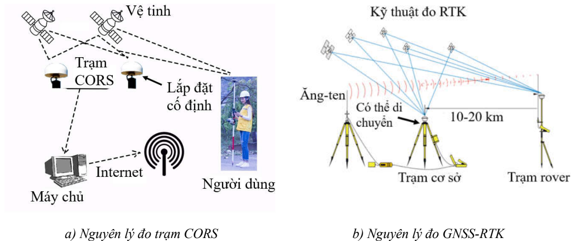
Hình 1. Nguyên lý đo CORS và GNSS-RTK.
